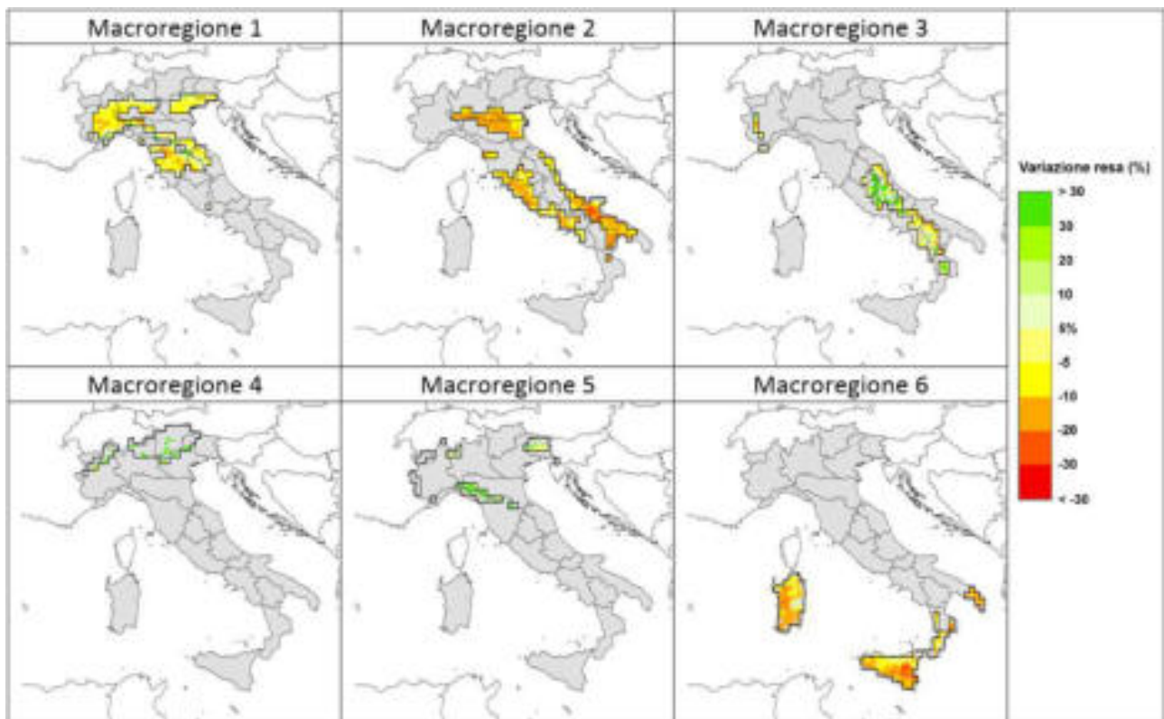
Figura 1-45: Proiezioni di variazione (%) di resa per il mais per le 6 zone climatiche in Italia, periodo 2021-2050, scenario RCP 8.5, modello climatico COSMO-CLM, a 8 km di risoluzione 79 .
