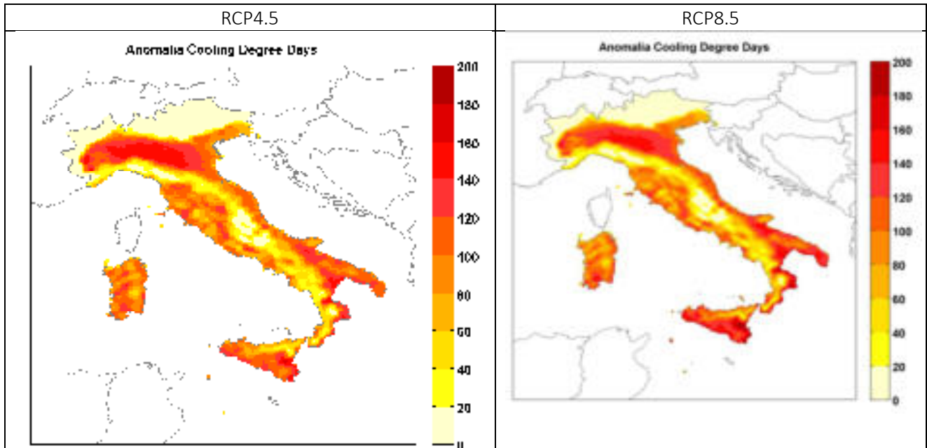
Figura 1-82: Anomalie medie annue di CDD per il trentennio 2011-2050 rispetto al trentennio di riferimento 1981-2010 (RCP4.5/RCP8.5). Fonte: CMCC, metodologia EUROSTAT/JRC.
